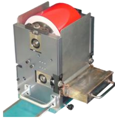
Printing unit Druckeinheit
