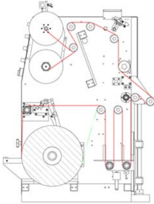
Layout Skizze
