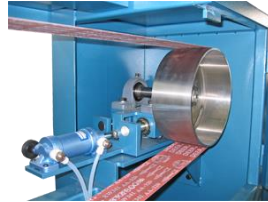
Automatic belt tension control Automatische Band Spannung
