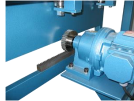
Drive for cart Antrieb für Transportwagen
