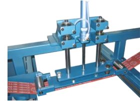
Pressure plate for sanding belt Anpressvorrichtung für Schleifband
