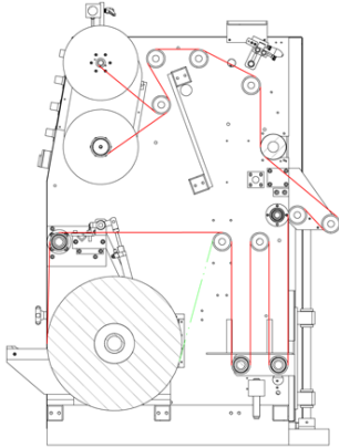
Layout Skizze
